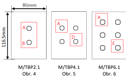
Obr. 4 – 6 Rozměry – čelní pohled
