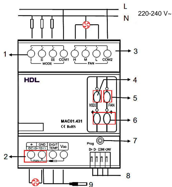
Zapojení HDL-MAC01.431
