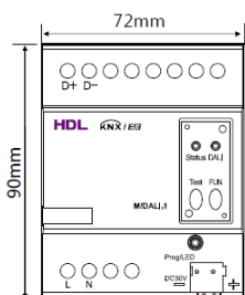
Obr. 2 Rozměry – čelní pohled
