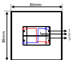
M/P02.2-48 Obr. 3 Rozměry – čelní pohled
