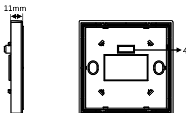
Figure 9. Dimensions - Side View Figure 10. Components - Back View 图 9. 尺寸图 - 侧面 图 10. 部件 - 背面图
