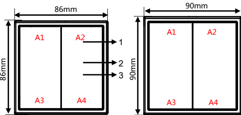
Figure 7. Dimensions - Plastic version Figure 8. Dimensions - Metal version 图 7. 尺寸图 - 塑料版本 图 8. 尺寸图 - 金属版本
